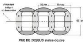
Pose des atalus-doubles
