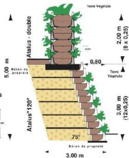
Coupe type Profil atalus double + atalus 120 0,95
