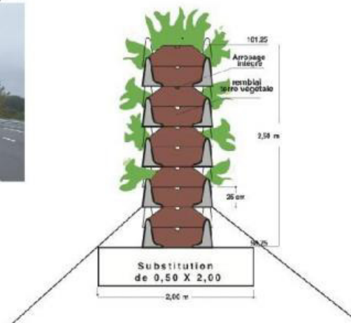
COUPE
