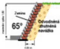
Příklady řezů
